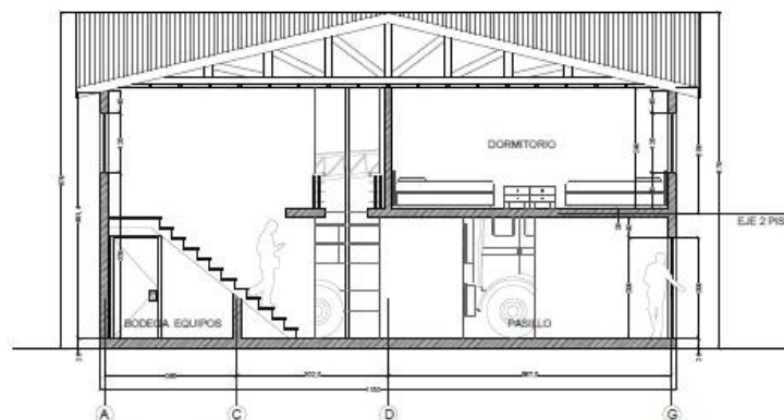
SECCIÓN b-b' ESCALA 1:50
