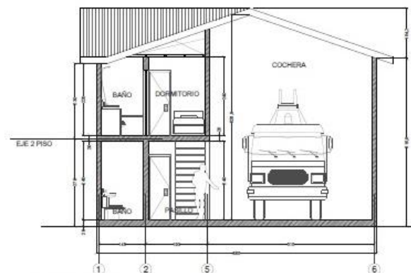
SECCIÓN a-a' ESCALA 1:50
