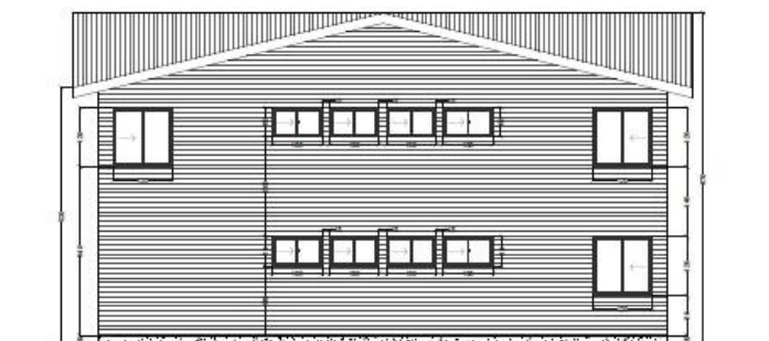
ELEVACIÓN SUR ESCALA 1:50
